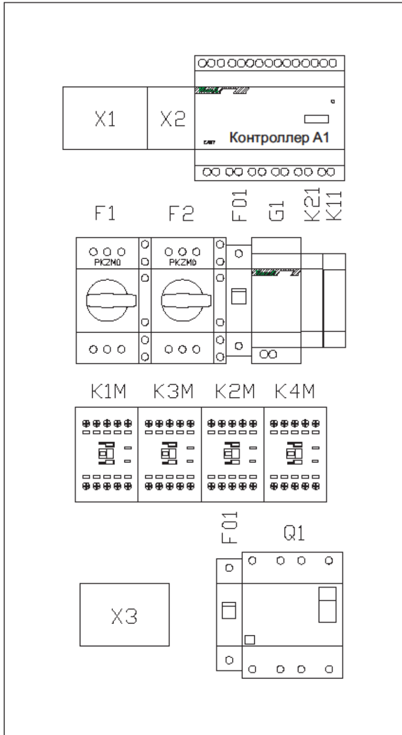
Расположение компонентов
